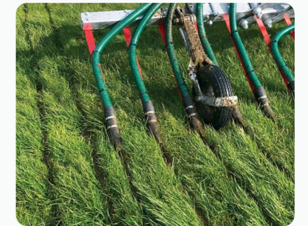
Rampe a patins en application de lisier en herbe longue et dense
